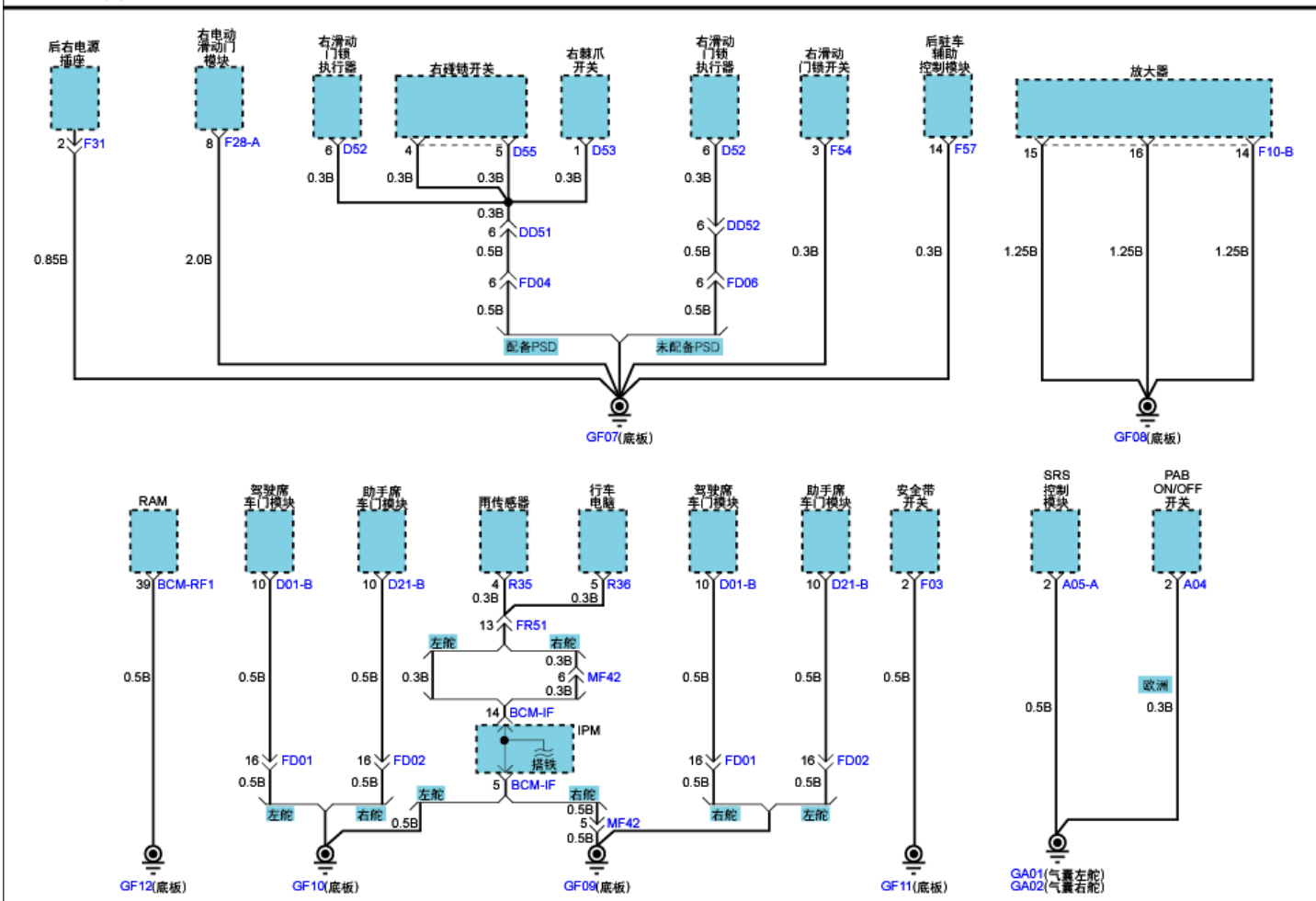
搭铁分布(8)
